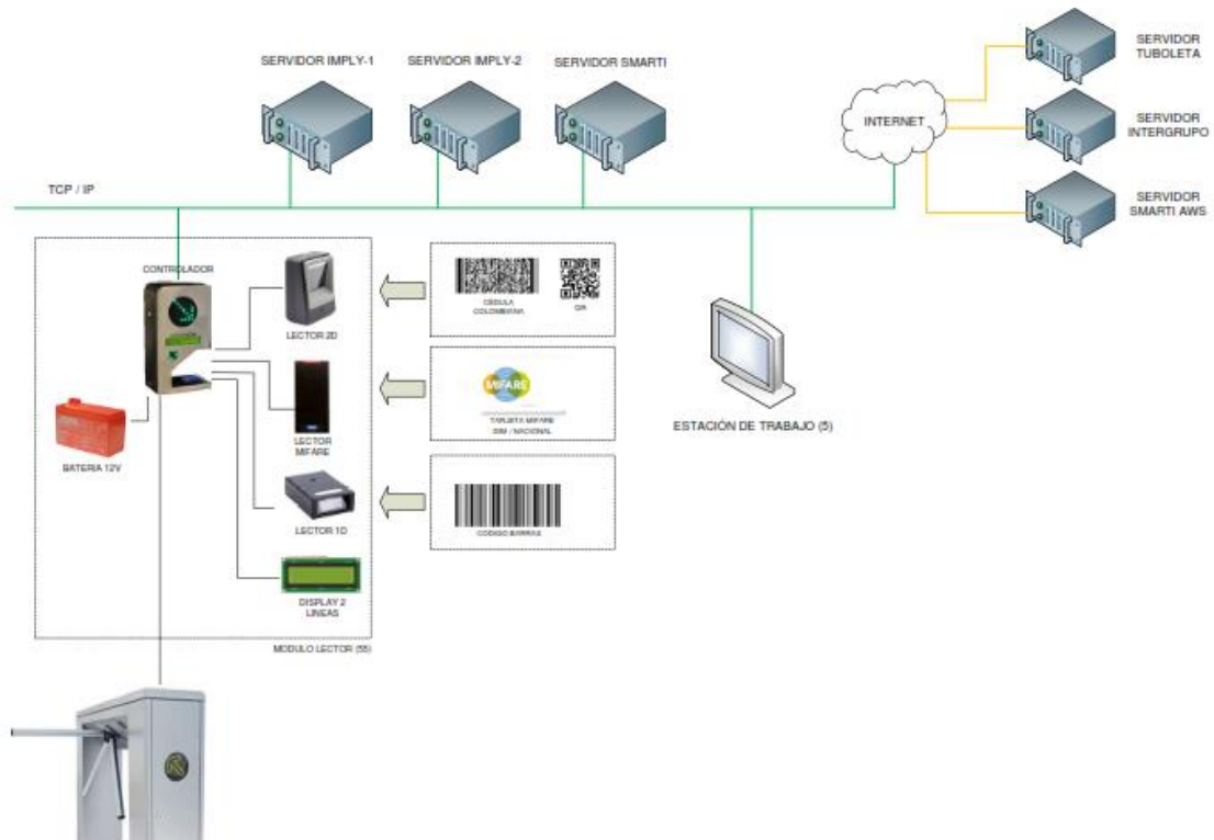
Ilustración 1 Arquitectura General
