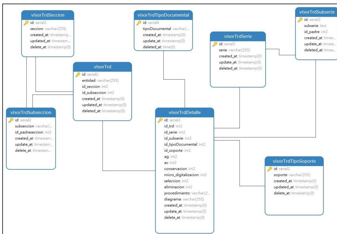
Figura 1. Estructura de la Base de Datos del Sistema de Información Visor 360
