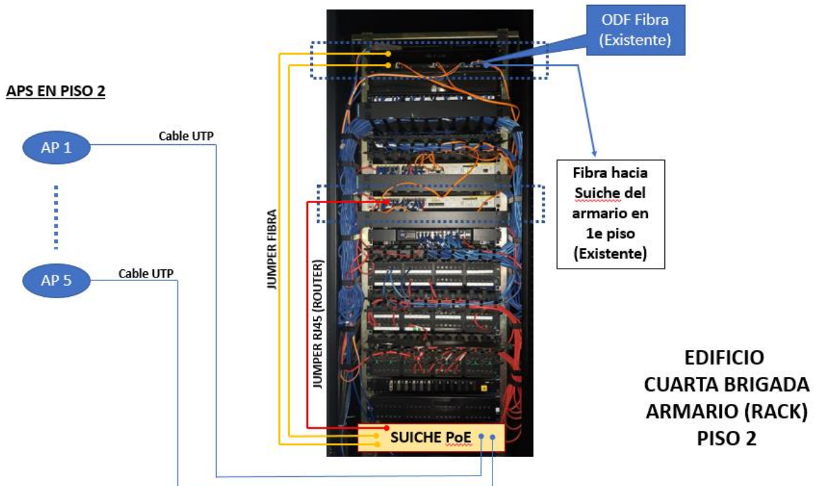
ILUSTRACIÓN 4. DIAGRAMA ESQUEMÁTICO DE CONEXIÓN PARA EL GABINETE DEL PISO 2
