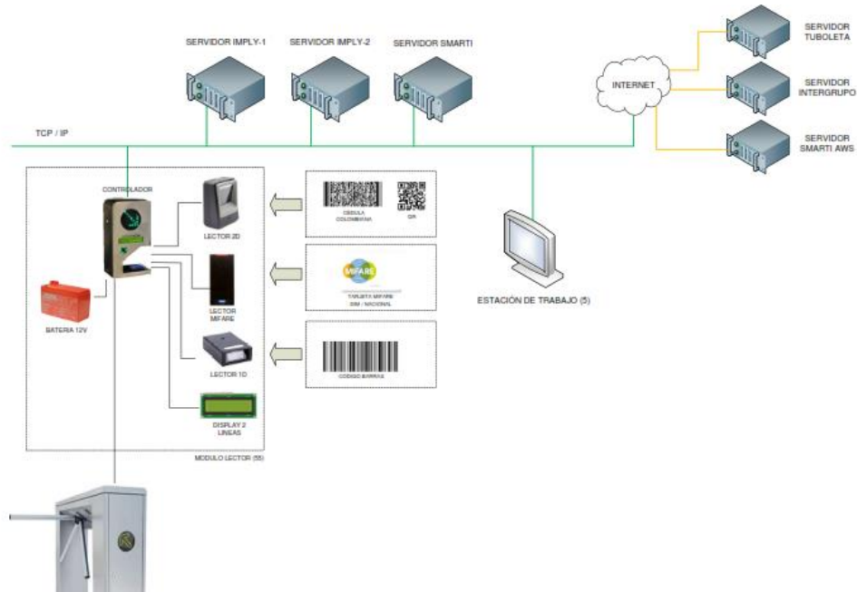
Ilustración 1 Arquitectura General
